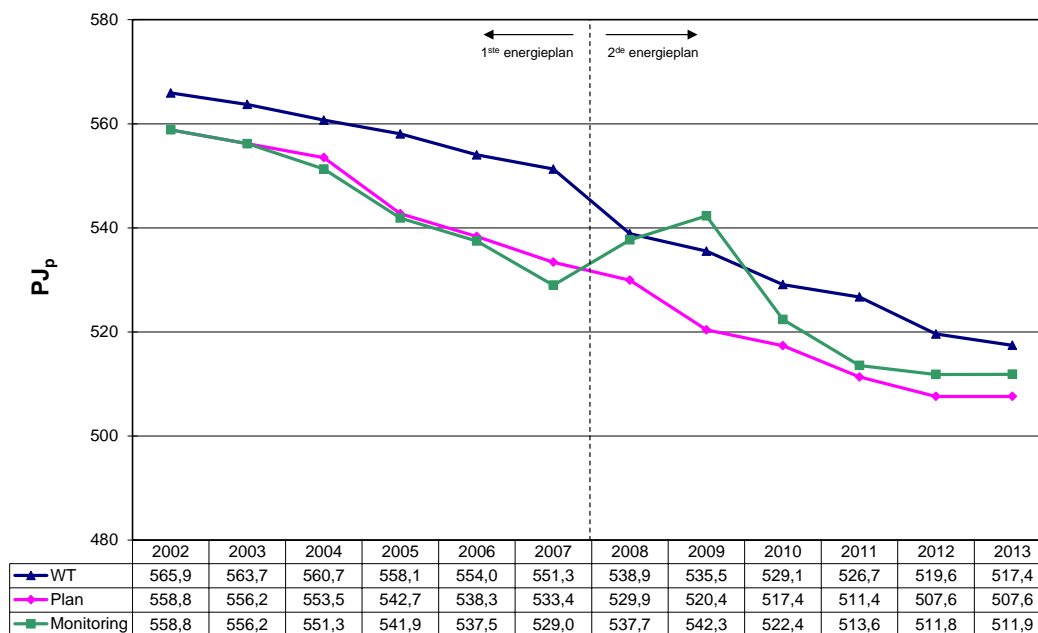
Figuur 3 : Evolutie primaire energieverbruik van alle bedrijven bij constante gerealiseerde productie 2013
