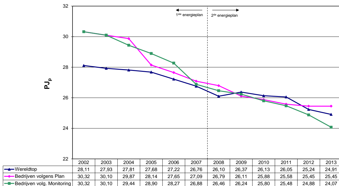
Figuur 11 : Evolutie primaire energieverbruik van de voedingsbedrijven bij constante gerealiseerde productie 2013
