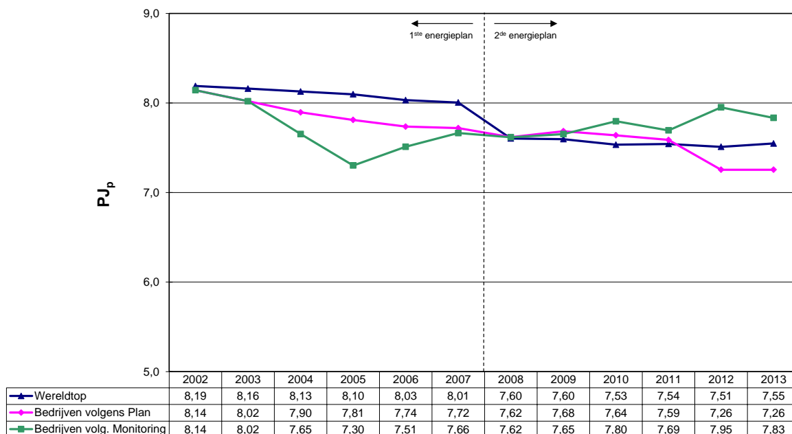
Figuur 21 : Evolutie primaire energieverbruik van de glasbedrijven, zandgroeven en diversen bij constante gerealiseerde productie 2013
