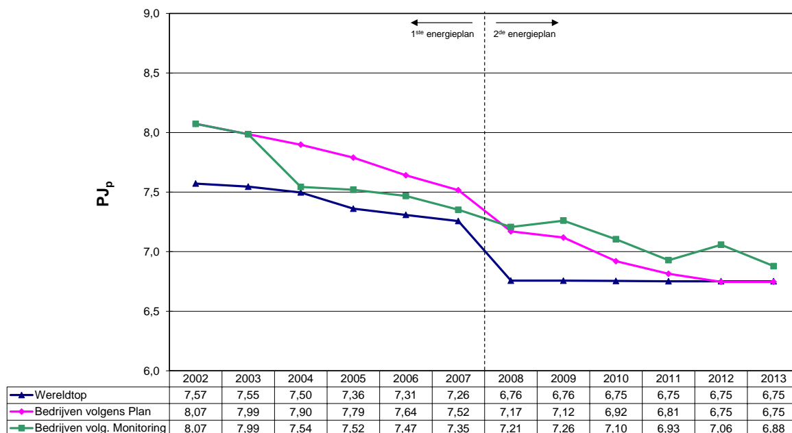
Figuur 15 : Evolutie primaire energieverbruik van de textielbedrijven bij constante gerealiseerde productie 2013
