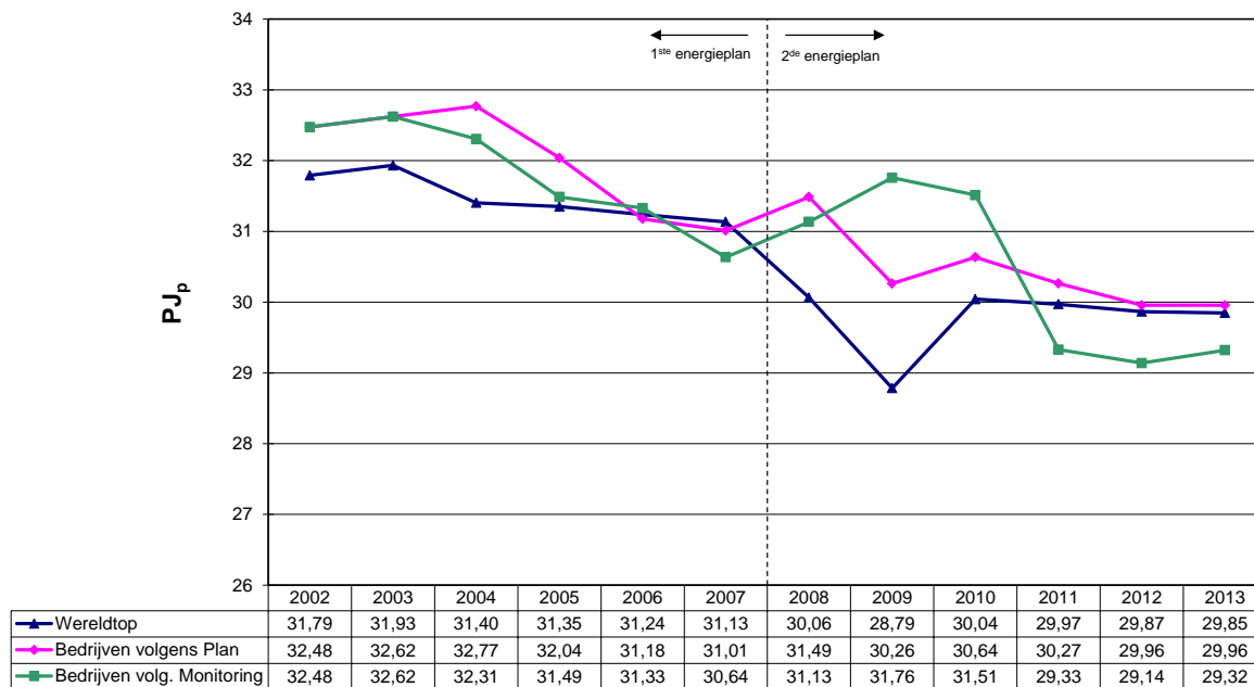
Figuur 13 : Evolutie primaire energieverbruik van de metaalbedrijven bij constante gerealiseerde productie 2013
