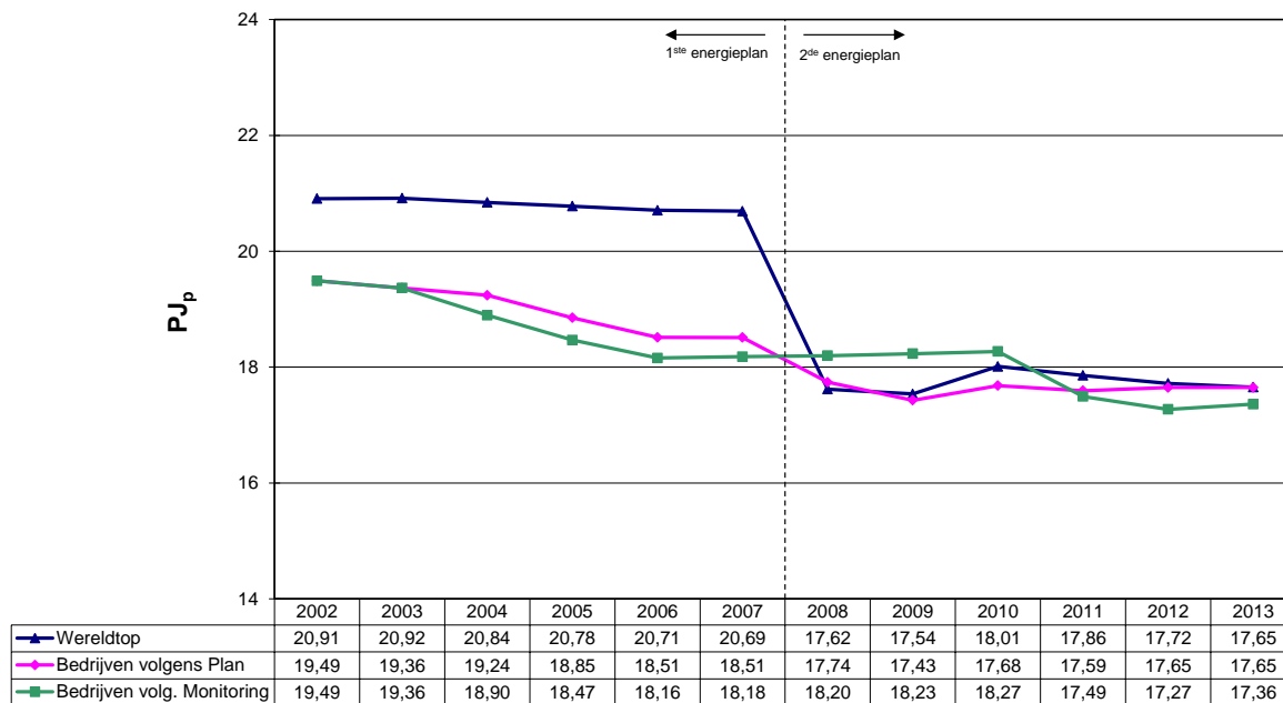
Figuur 9 : Evolutie primaire energieverbruik van de papierbedrijven bij constante gerealiseerde productie in 2013
