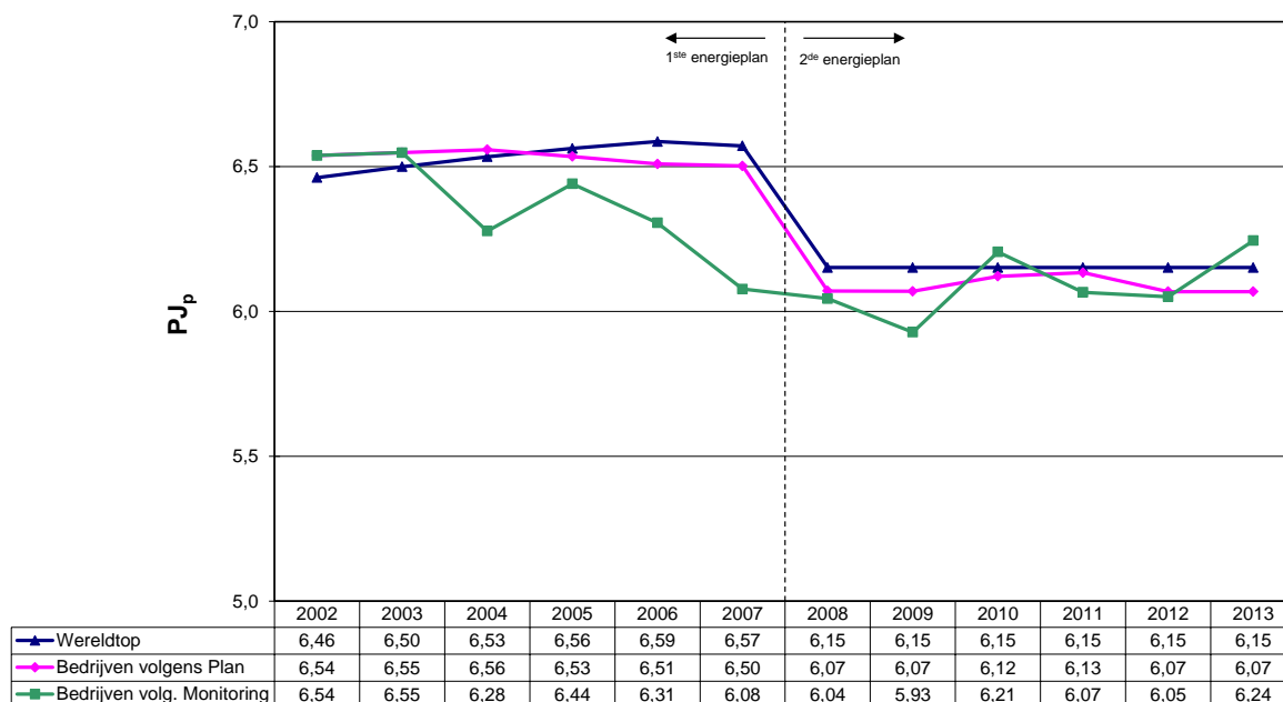
Figuur 17 : Evolutie primaire energieverbruik van de keramische sector bij constante gerealiseerde productie 2013
