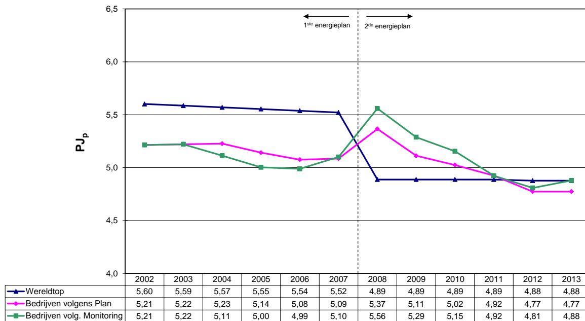
Figuur 19 : Evolutie primaire energieverbruik van de houtspaanbedrijven bij constante gerealiseerde productie 2013
