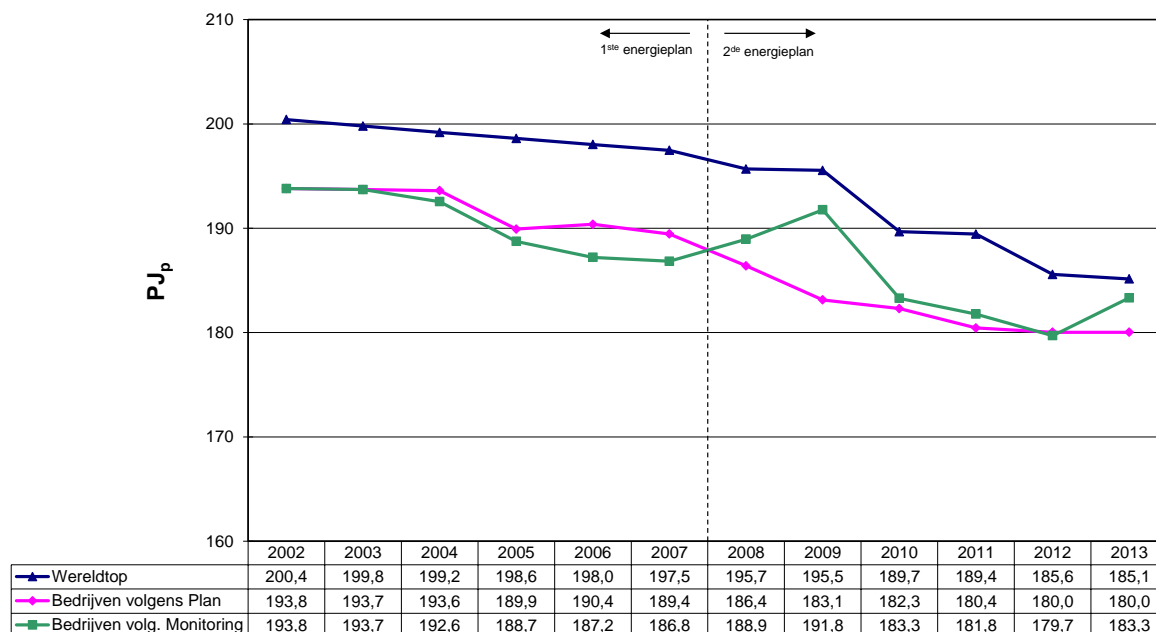
Figuur 7 : Evolutie primaire energieverbruik van de raffinaderijen en staalbedrijven bij constante gerealiseerde productie 2013
