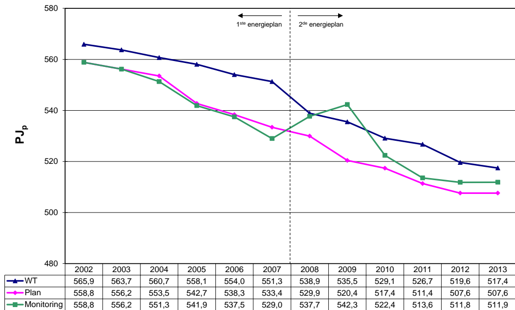
Figuur 1: Evolutie primaire energieverbruik van alle bedrijven bij constante gerealiseerde productie 2013
